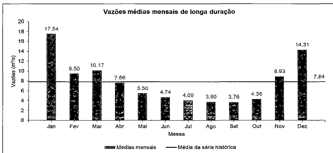
Figura 3-22 - Gráfico das vazões médias de longa duração para a estação Afonso Cláudio – Montante.
