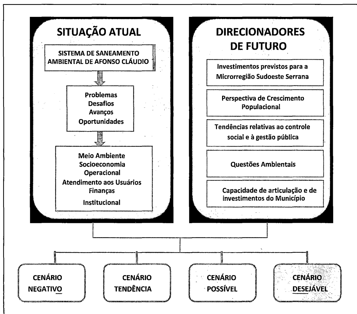
Figura 4-1 - Esquema metodológico.
