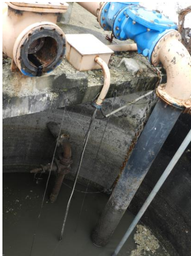
Figura 21 - Ausência de bomba reserva na EEEB Maria Ortiz.
