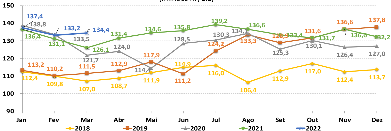
Produção Diária - Espírito Santo (milhões m 3 /dia)
