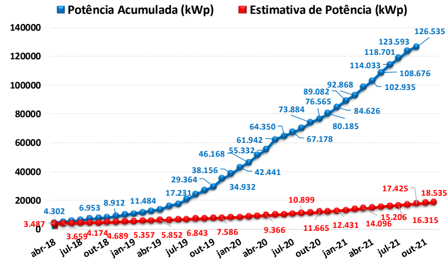
Potência Instalada em Microgeração no ES - kWp
