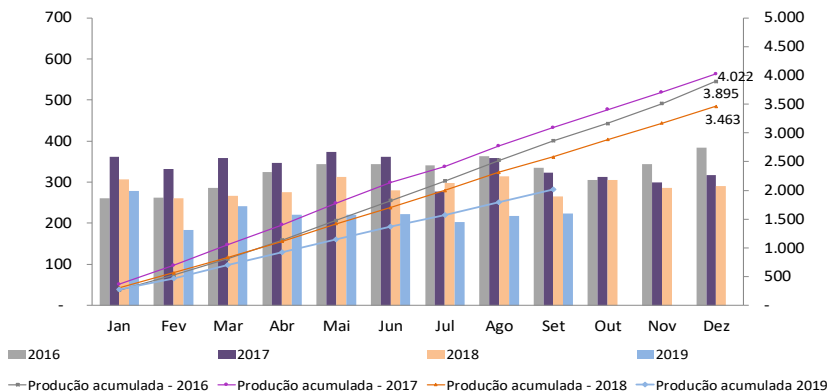
Produção Mensal – Espírito Santo (milhões m 3 )
