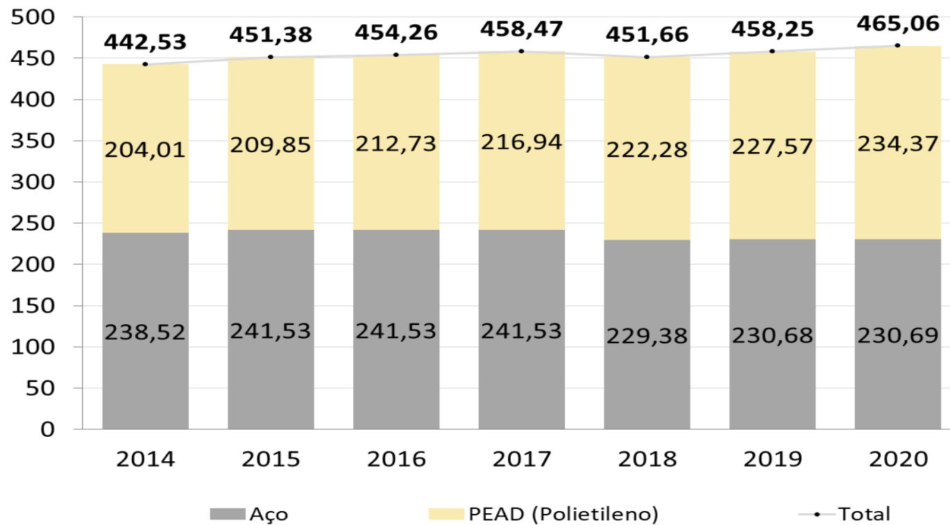
Evolução da Rede de Distribuição por Material (km)
