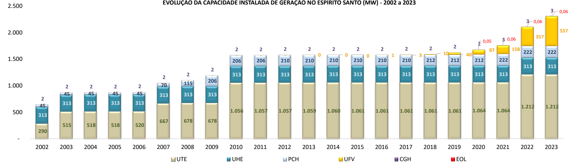
EVOLUÇÃO DA CAPACIDADE INSTALADA DE GERAÇÃO NO ESPÍRITO SANTO (MW) - 2002 a 2023
