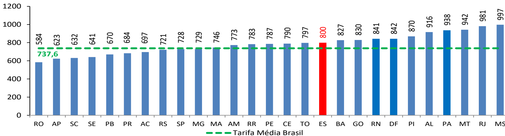
Tarifa Média Industrial com Tributos (R$/MWh)
