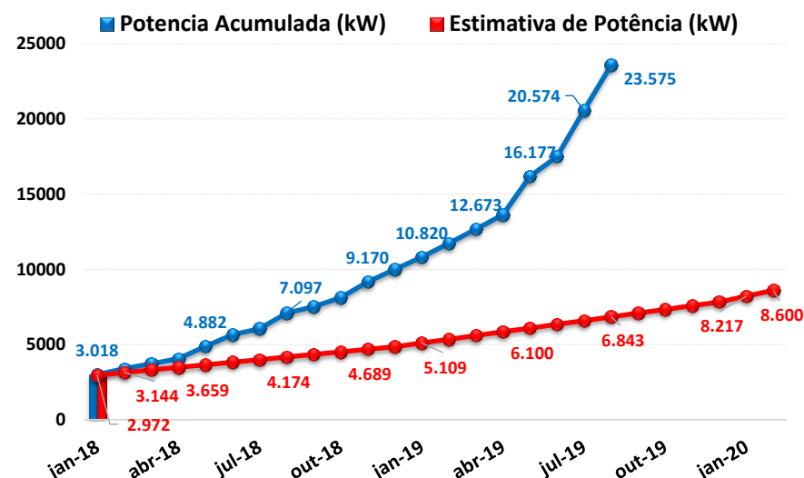
Potência Instalada em Microgeração no ES - kW
