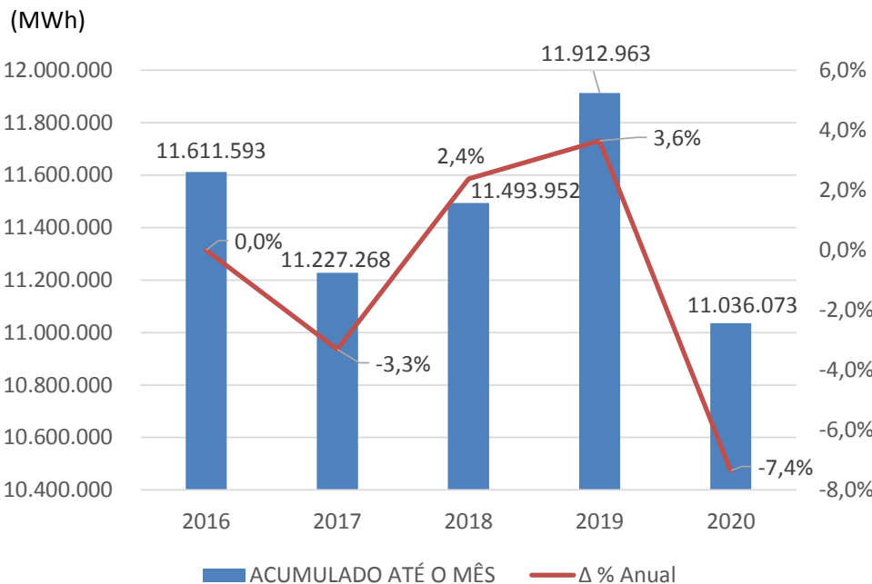
ACUMULADO DE ENERGIA DISTRIBUÍDA (MWh)
