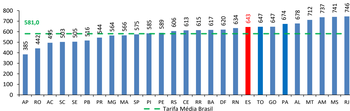
Tarifa Média Industrial sem Tributos (R$/MWh)
