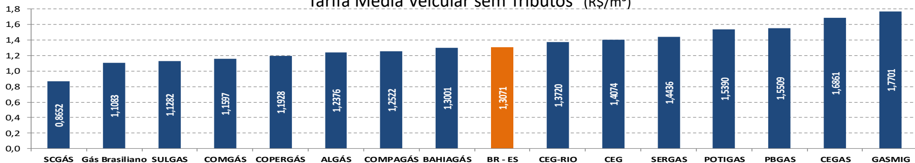
Tarifa Média Veicular sem Tributos 3 (R$/m 3 )
