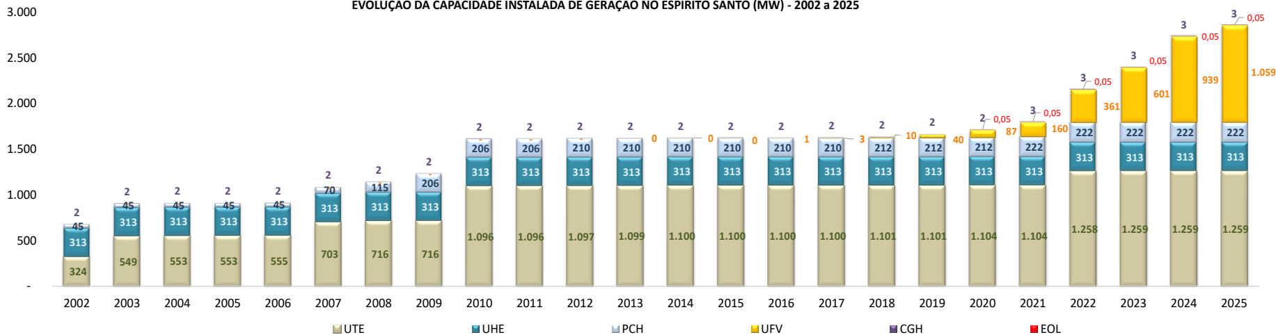
EVOLUÇÃO DA CAPACIDADE INSTALADA DE GERAÇÃO NO ESPÍRITO SANTO (MW) - 2002 a 2025
