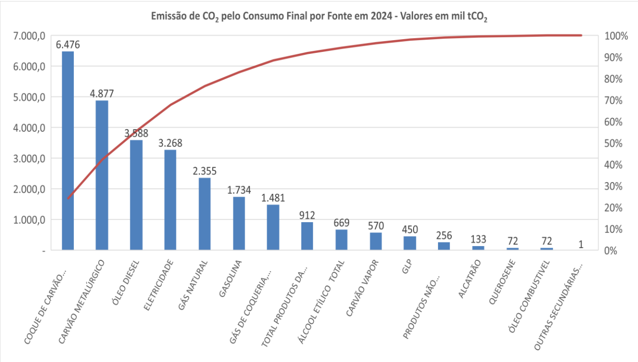
Gráfico 6.4.1 - Emissão de CO 2 pelo Consumo Final por Fonte no ES, em 2024 - Valores em mil tCO 2 Graph 6.4.1 - CO 2 Emission by Final Consumption by Source in ES, in 2024 - Values in thousand tCO 2
