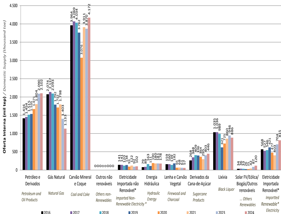
Gráfico 4.1.2 - Oferta Interna Bruta Energética no Espírito Santo por Fonte Graph 4.1.2 - Gross Domestic Energetic Supply in Espírito Santo by Source
