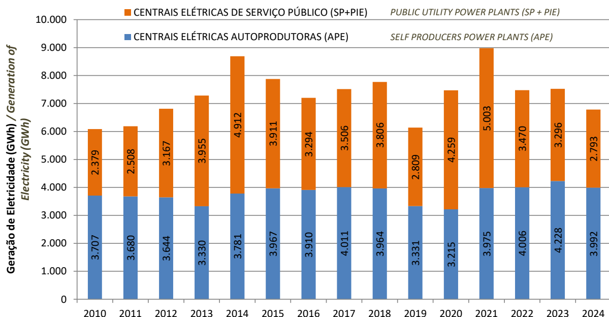
Gráfico 8.1.1 - Evolução da Geração de Energia Elétrica Autoprodução X Serviço Público no ES Graph 8.1.1 - Evolution of Electric Power Generation - Self-production X Public Service in the ES
