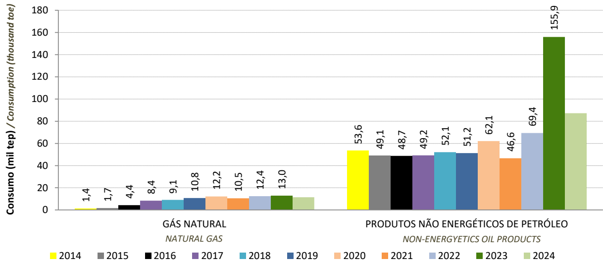
Gráfico 6.2.3 - Consumo Final Não Energético no ES por Fonte - Valores em mil tep Graph 6.2.3 - Non-Energetic Final Consumption in ES by Source - Values in thousand toe
