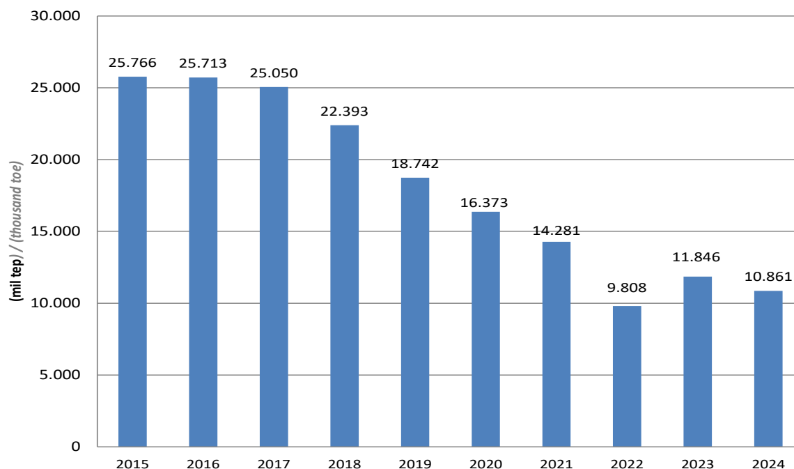
Gráfico 3.1.1 - Produção Energética no Espírito Santo – Valores em mil tep Graph 3.1.1 - Energetic Production in Espírito Santo - Values in thousand toe
