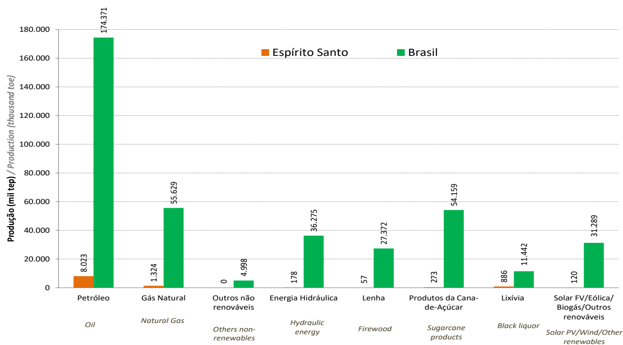
Gráfico 3.1.2 – Comparação da Produção Energética Espírito Santo X Brasil – 2024 Graph 3.1.2 - Comparison of Energy Production Espírito Santo X Brazil - 2024
