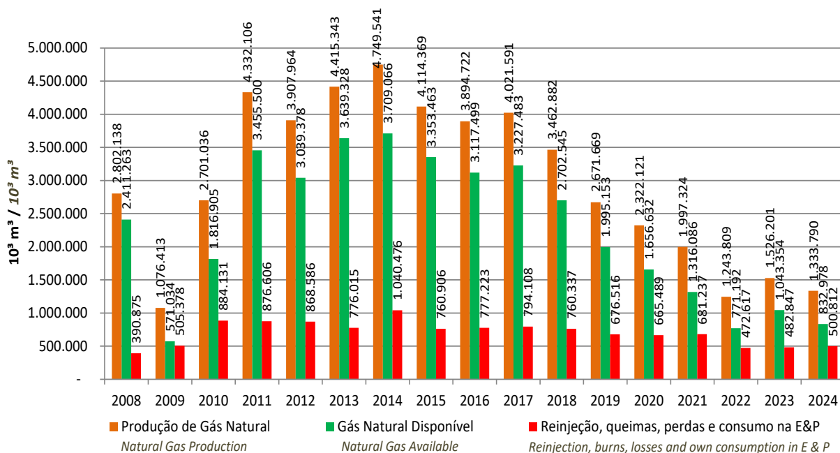
Gráfico 7.2.1.1 - Evolução da Produção* de Gás Natural no Espírito Santo - Valores em 10 3 m 3 Graph 7.2.1.1 - Evolution of Natural Gas Production* in Espírito Santo - Values in 10 3 m 3
