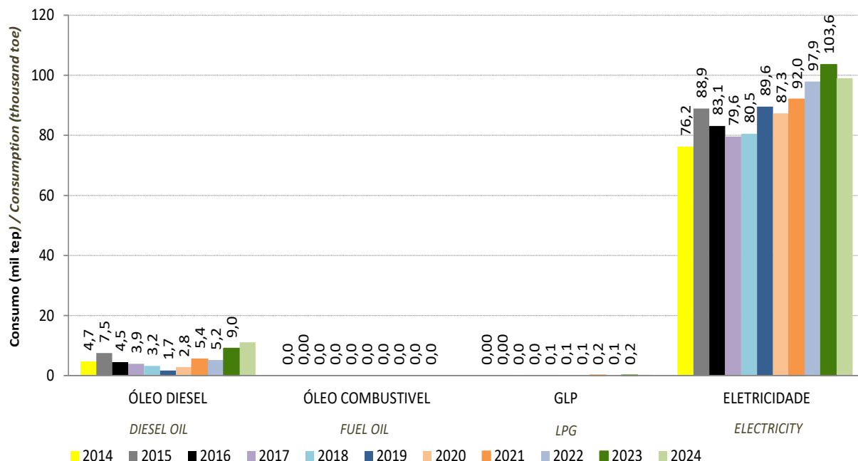
Gráfico 6.2.8 - Consumo Final Setor Agropecuário no ES por Fonte - Valores em mil tep Graph 6.2.8 - Final Consumption of the Agriculture and Livestock Sector in ES by Source - Values in thousand toe
