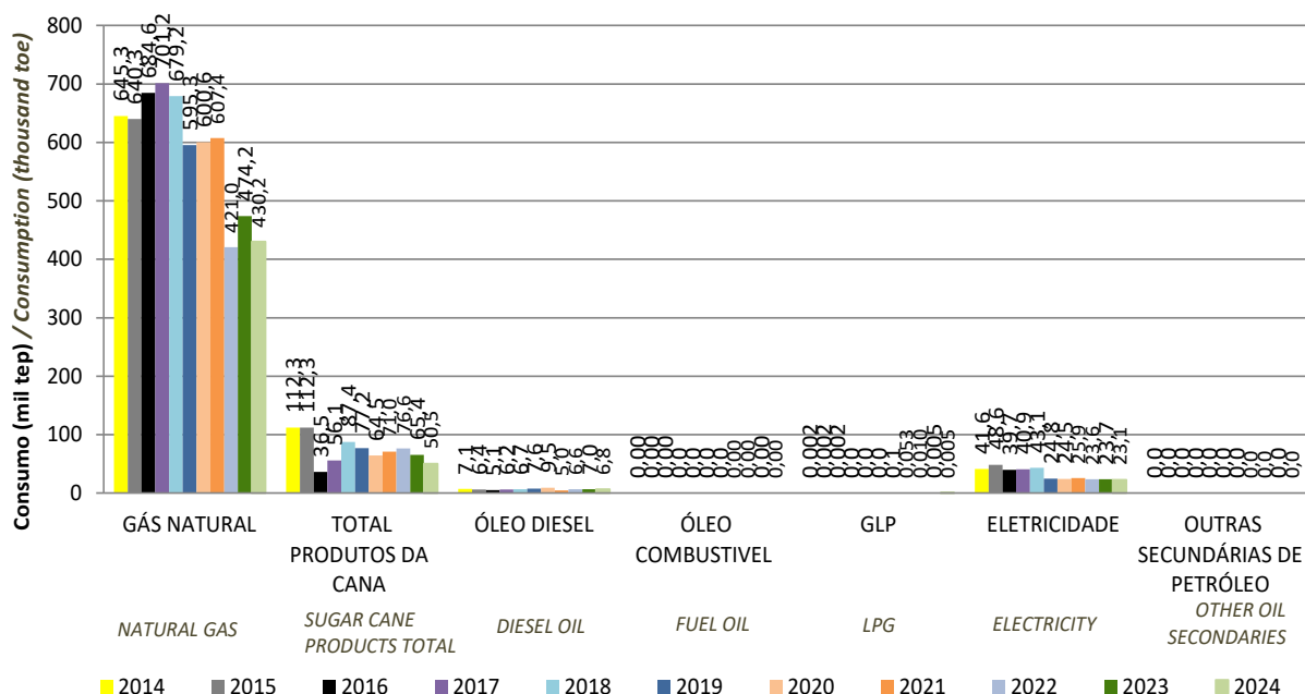
Gráfico 6.2.4 - Consumo Final Setor Energético no ES por Fonte - Valores em mil tep Graph 6.2.4 - Final Consumption Energetic Sector in ES by Source - Values in thousand toe
