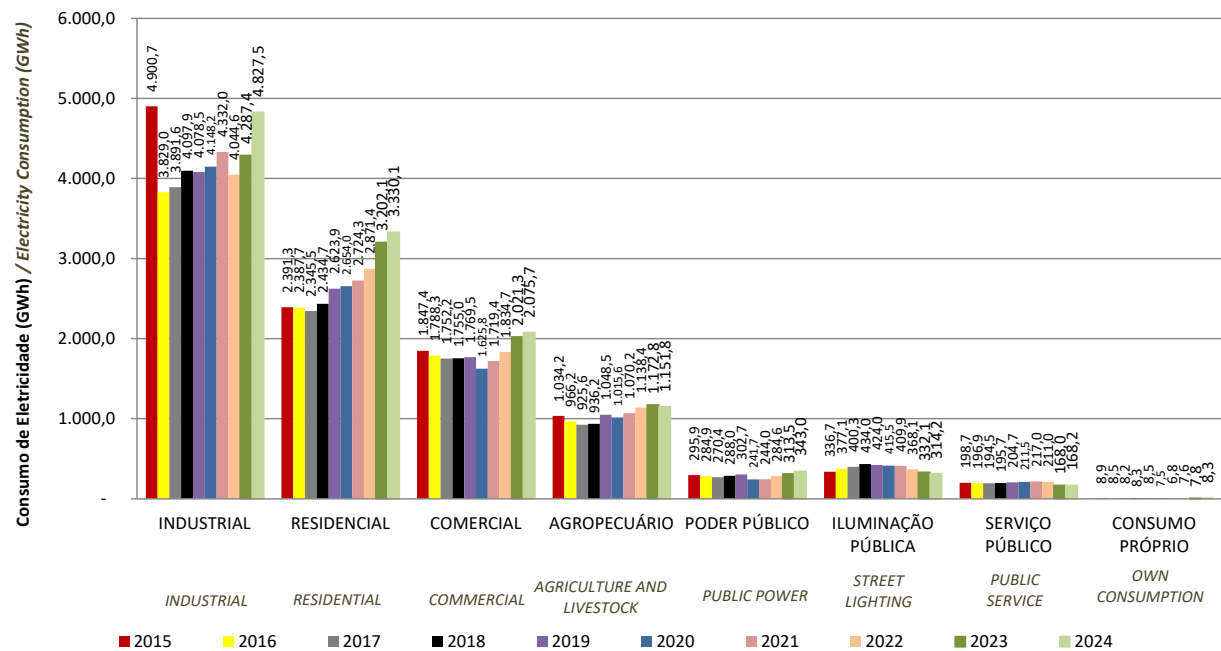
Gráfico 8.2.5 - Evolução do Consumo da Energia Elétrica Distribuída - Valores em GWh Graph 8.2.5 - Evolution of Electricity Consumption Distributed - Values in GWh
