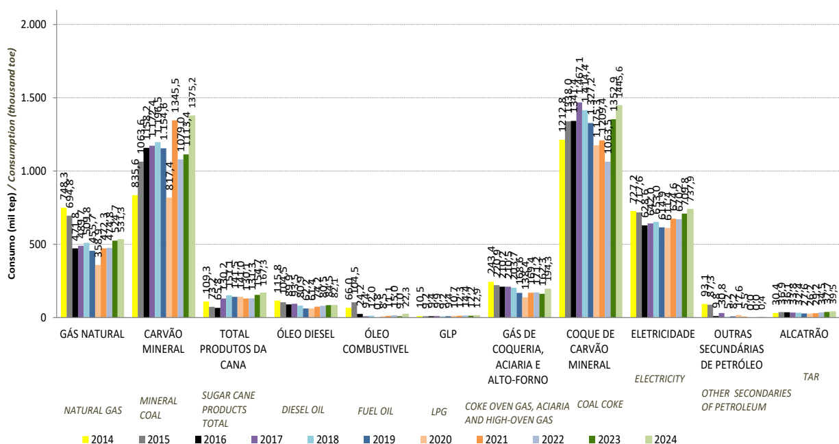
Gráfico 6.2.10 - Consumo Final Setor Industrial no ES por Fonte - Valores em mil tep Graph 6.2.10 - Final Consumption of Industrial Sector in ES by Source - Values in thousand toe
