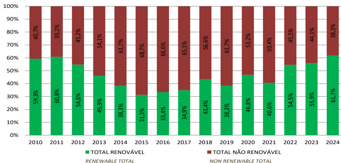
Gráfico 8.1.2 - Evolução da Geração de Energia Elétrica Renovável X Não Renovável no ES Graph 8.1.2 - Evolution of Electric Power Generation Renewable X Non-renewable in the ES
