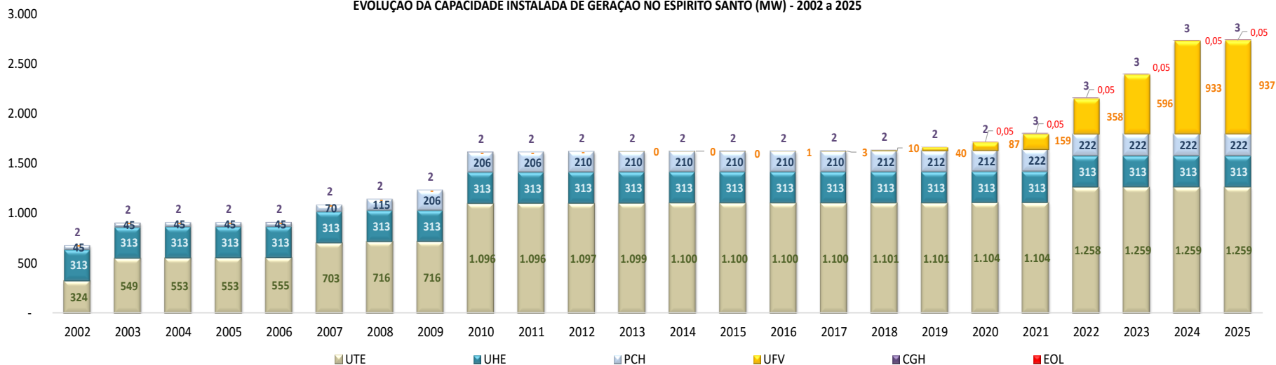
EVOLUÇÃO DA CAPACIDADE INSTALADA DE GERAÇÃO NO ESPÍRITO SANTO (MW) - 2002 a 2025
