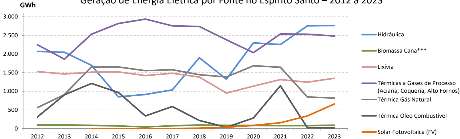
Geração de Energia Elétrica por Fonte no Espírito Santo – 2012 a 2023
