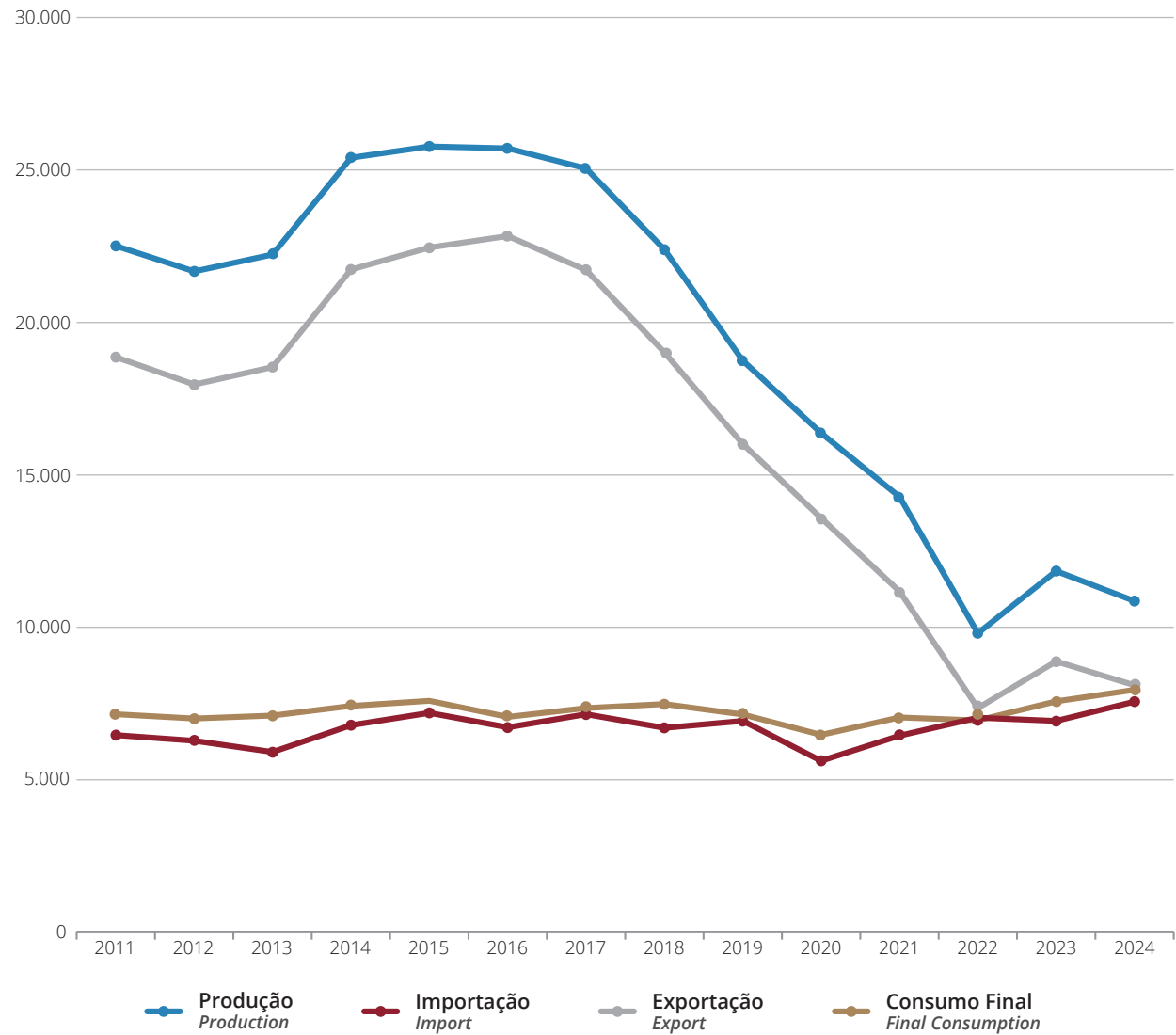
Gráfico 2.1.1 - Evolução do Fluxo Energético do Espírito Santo - Valores em mil tep Graph 2.1.1 - Evolution of the Espírito Santo Energetic Flow - Values in thousand toe
