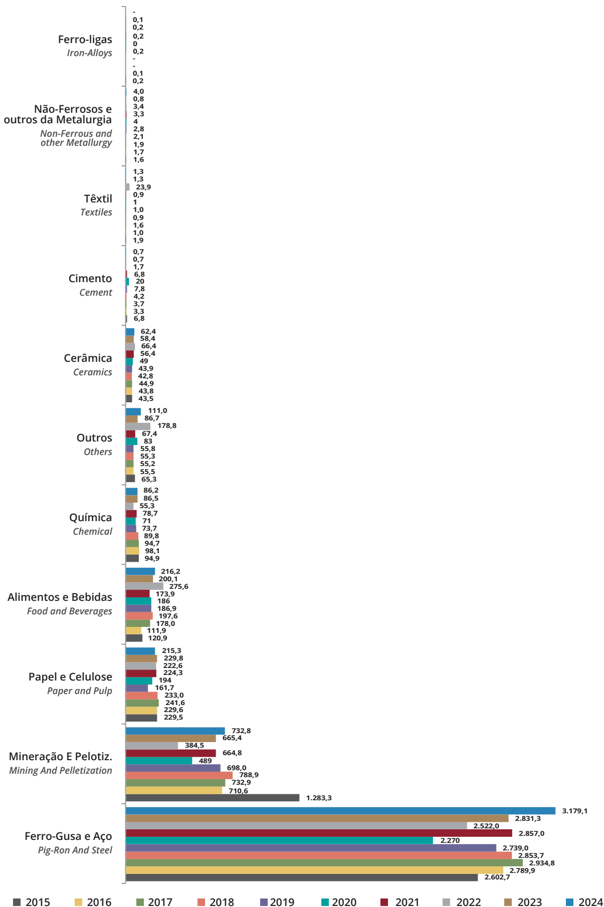
Gráfico 6.3.1 - Consumo Final Setor Industrial no ES por Ramo de Atividade - Valores em mil tep
