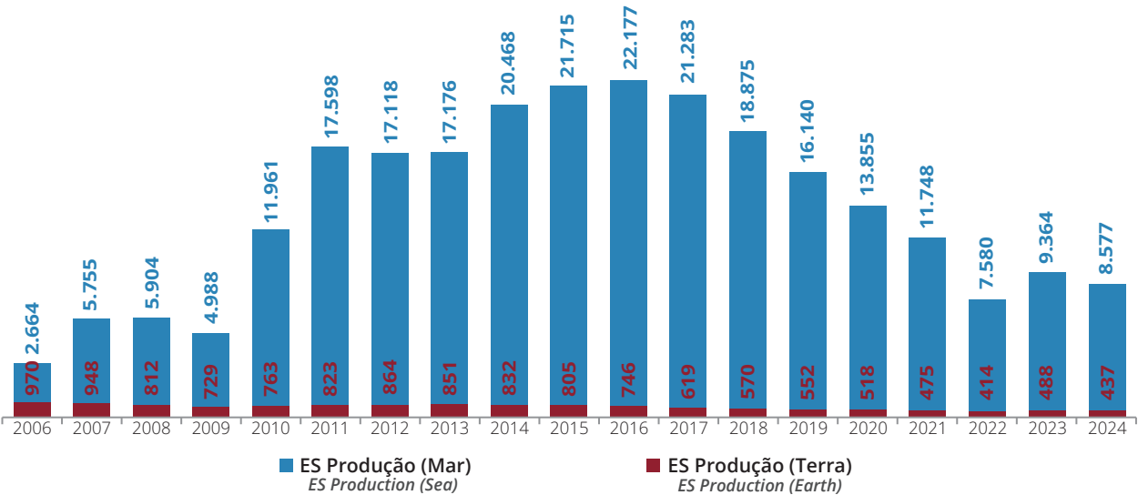
Gráfico 7.1.1 - Produção de Petróleo no Espírito Santo - Valores em 10³ m³ Graph 7.1.1 - Petroleum Production in Espírito Santo - Values in 10³ m³
