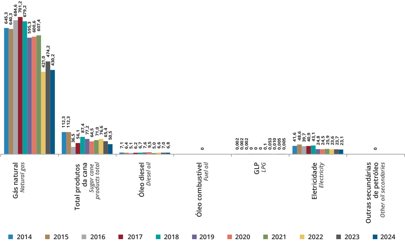
Gráfico 6.2.4 - Consumo Final Setor Energético no ES por Fonte - Valores em mil tep Graph 6.2.4 - Final Consumption Energetic Sector in ES by Source - Values in thousand toe
