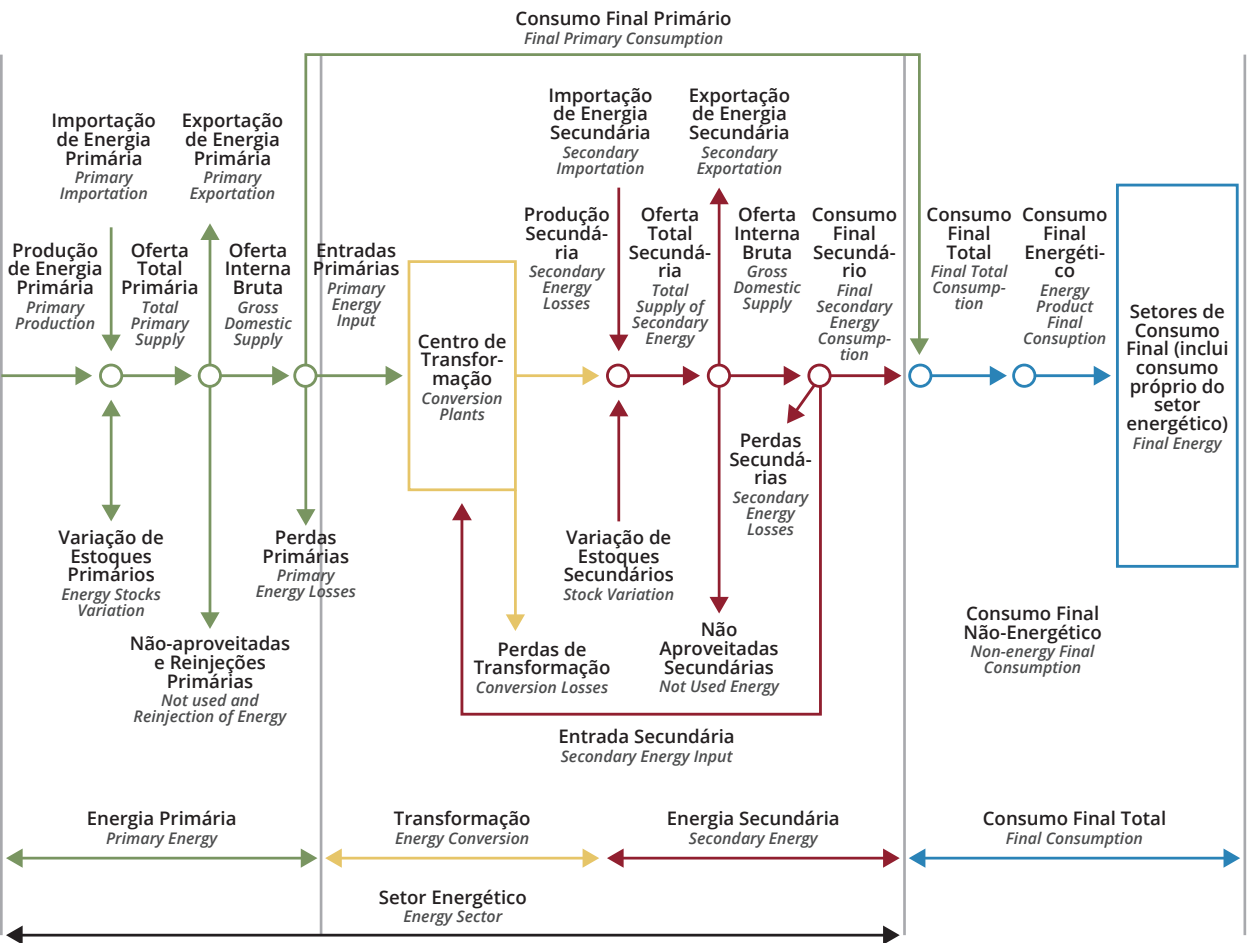
Figura 10.1.1 - Estrutura dos Fluxos de Energia do Balanço Estadual Figure 10.1.1 - General Structure of the State of the Espírito Santo Energy Balance
