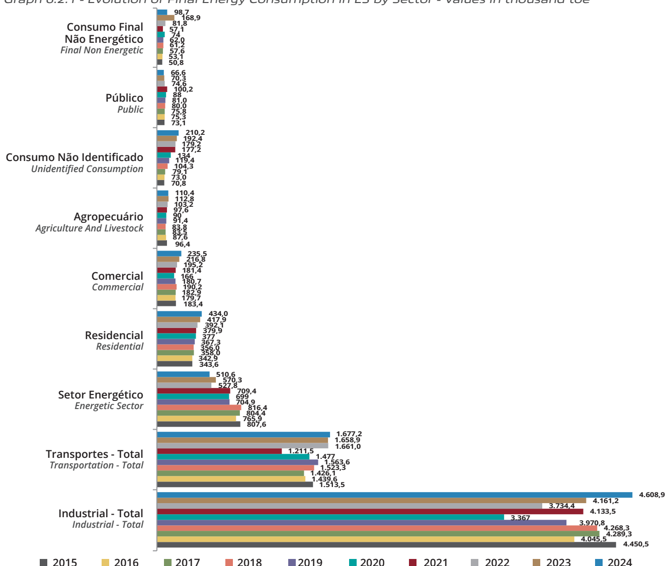
Gráfico 6.2.1 – Evolução do Consumo Final Energético no ES por Setor – Valores em mil tep Graph 6.2.1 - Evolution of Final Energy Consumption in ES by Sector - Values in thousand toe
