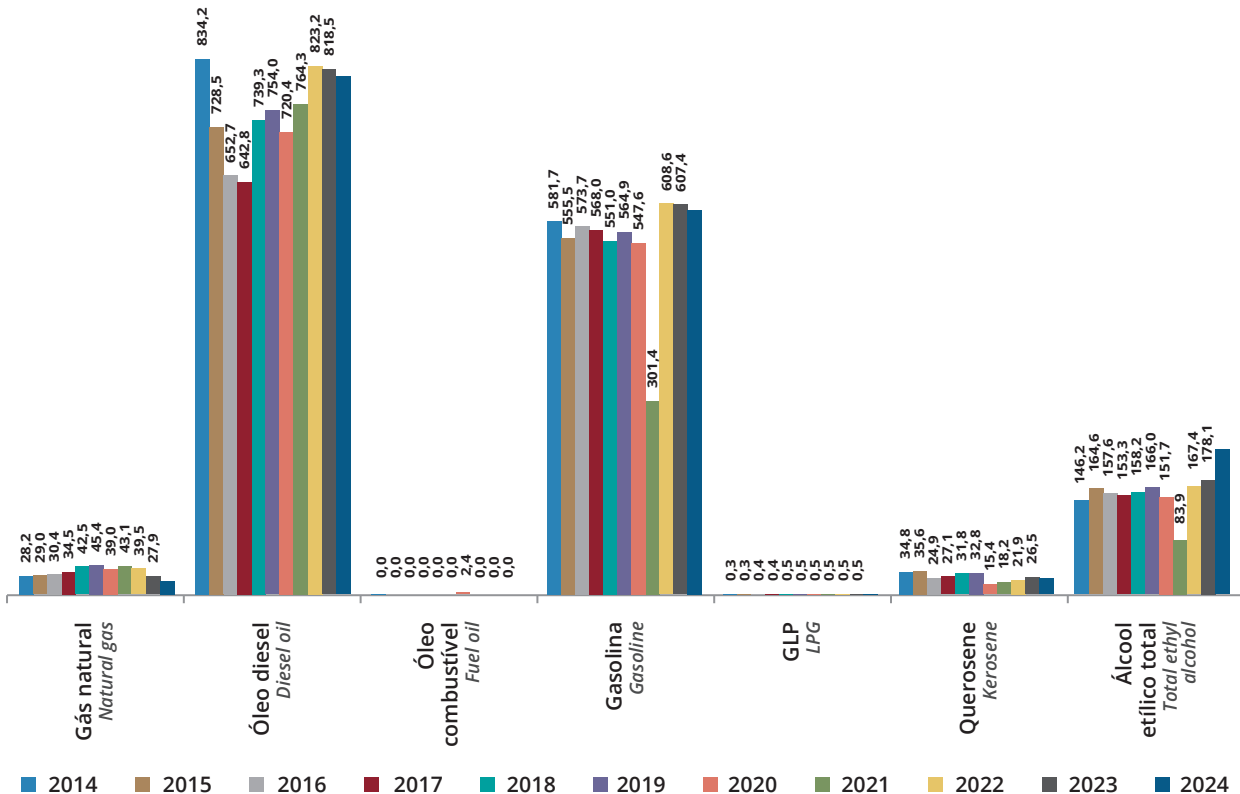
Gráfico 6.2.9 - Consumo Final Setor de Transporte no ES por Fonte - Valores em mil tep Graph 6.2.9 - Final Consumption of the Transportation Sector in ES by Source - Values in thousand toe
