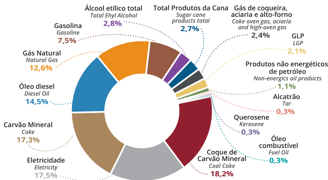
Gráfico 6.1.3 – Distribuição por Fonte do Consumo Final Energético no Espírito Santo – 2024 Graph 6.1.3 - Distribution by Source of Energetic Final Consumption in Espírito Santo – 2024
