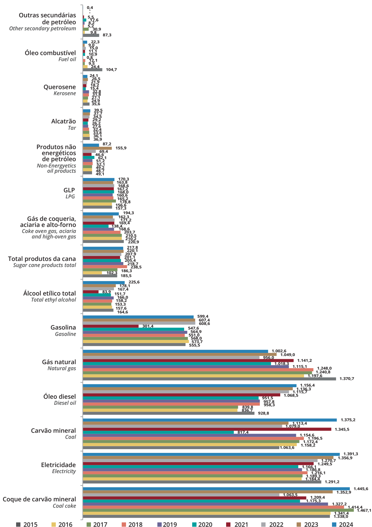
Gráfico 6.1.2 - Evolução do Consumo Final Energético no Espírito Santo por Fonte – Valores em mil tep Graph 6.1.2 - Evolution of Energetic Final Consumption in Espírito Santo by Source - Values in thousand toe
