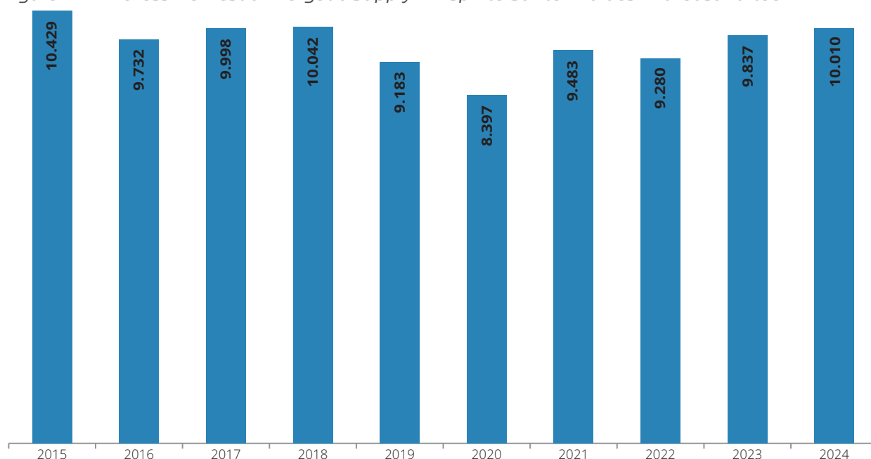
Gráfico 4.1.1 - Oferta Interna Bruta Energética no Espírito Santo - Valores em mil tep
