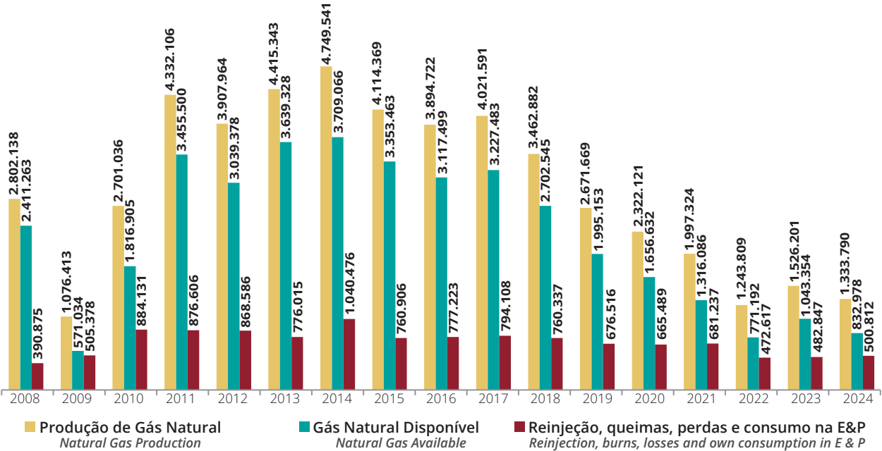
Gráfico 7.2.1.1 - Evolução da Produção* de Gás Natural no Espírito Santo - Valores em 10³m³ Graph 7.2.1.1 - Evolution of Natural Gas Production* in Espírito Santo - Values in 10³m³
