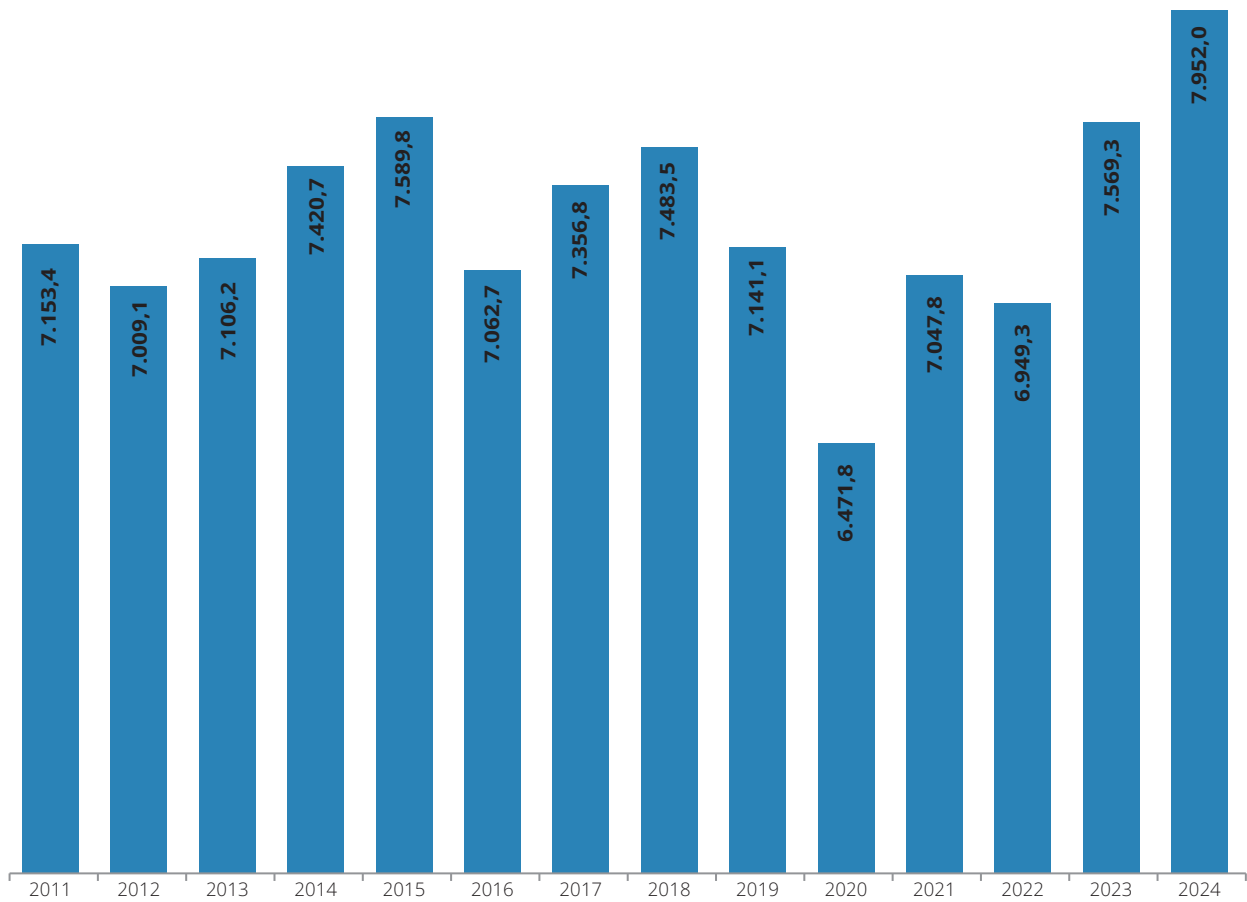
Gráfico 6.1.1 - Evolução do Consumo Final Energético no Espírito Santo – Valores em mil tep Graph 6.1.2 - Evolution of Energetic Final Consumption in Espírito Santo - Values in thousand toe
