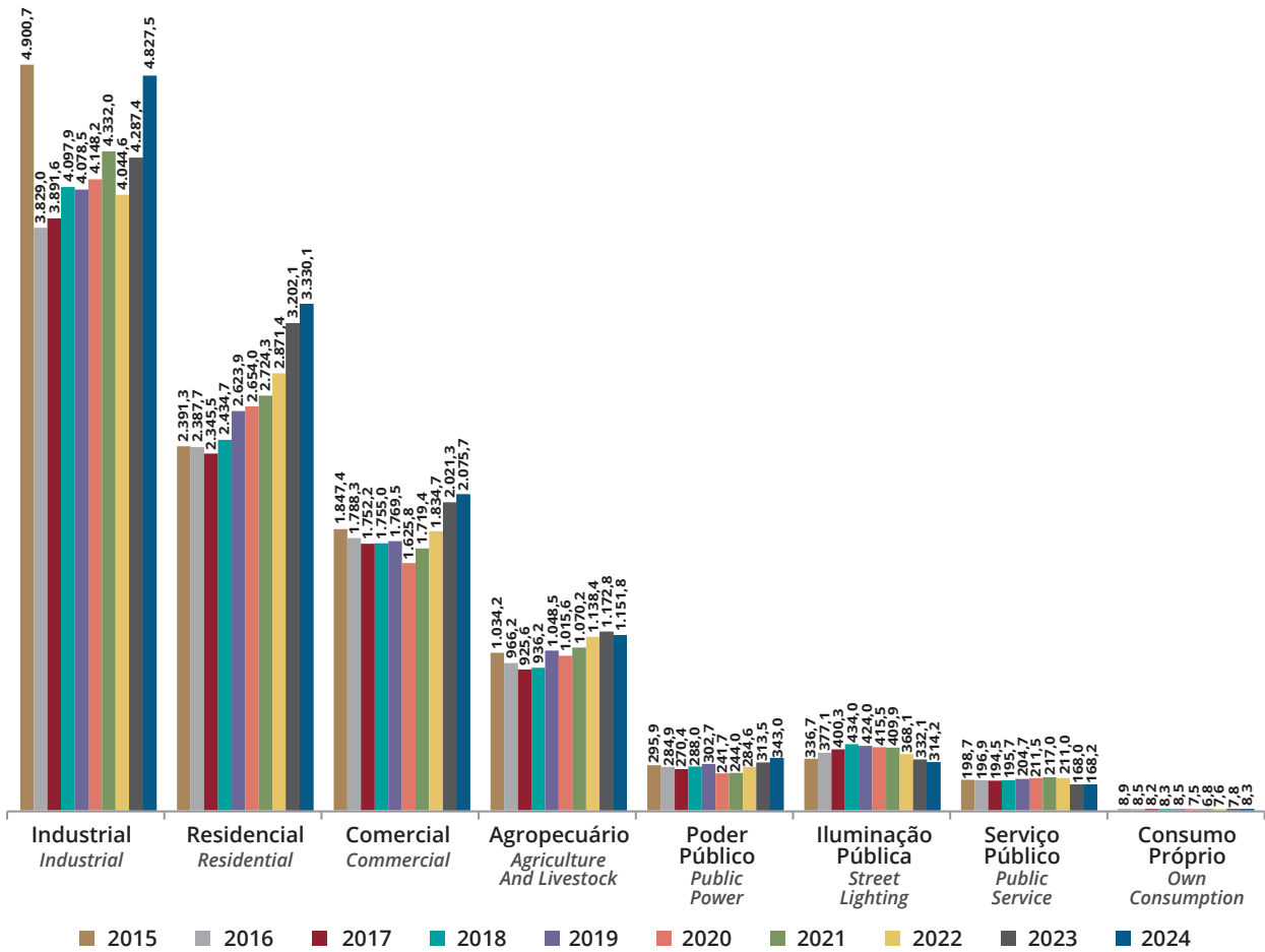
Gráfico 8.2.5 - Evolução do Consumo da Energia Elétrica Distribuída - Valores em GWh Graph 8.2.5 - Evolution of Electricity Consumption Distributed - Values in GWh
