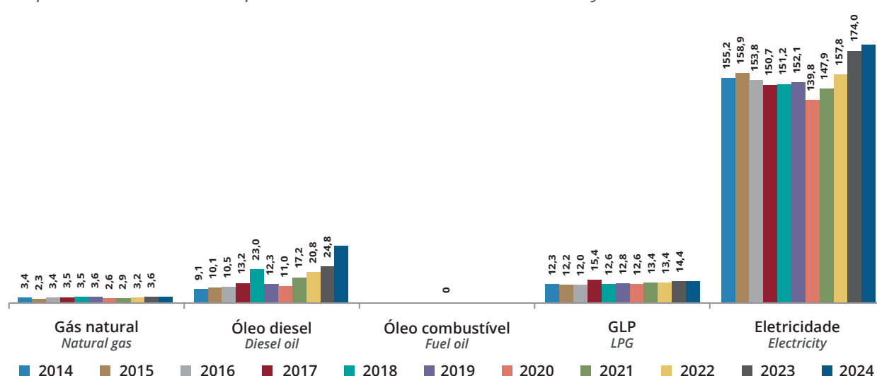
Gráfico 6.2.6 - Consumo Final do Setor Comercial no Espírito Santo por Fonte - Valores em mil tep
