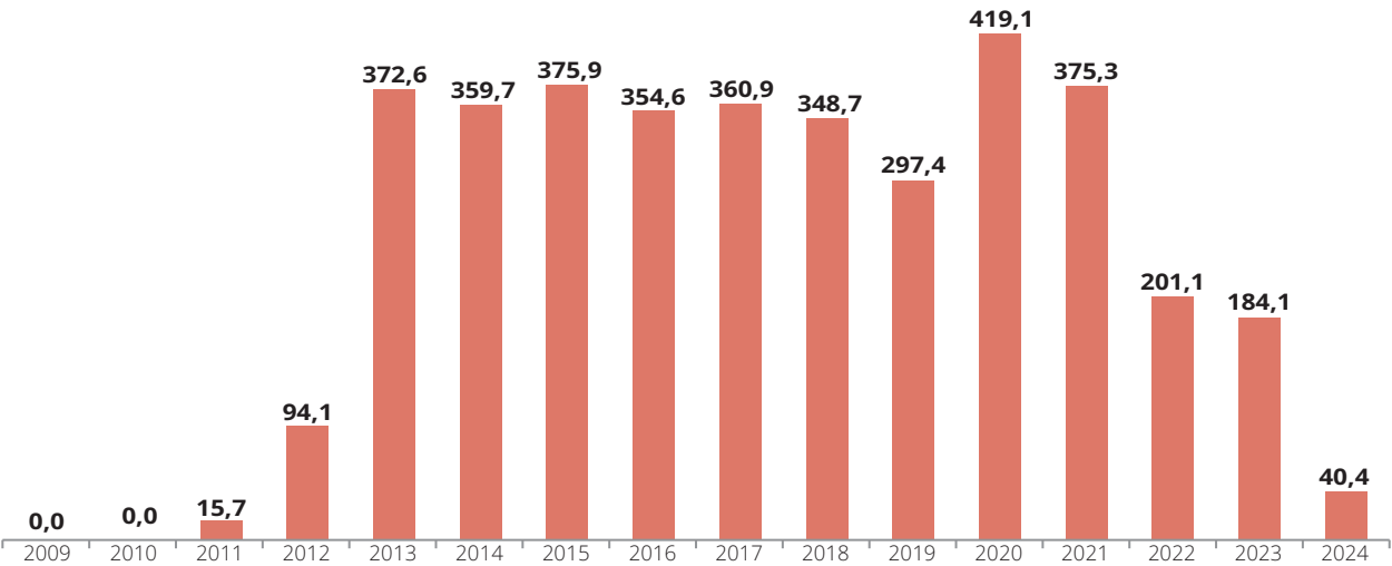
Gráfico 7.2.2.3 - Evolução do Consumo de Gás Natural em Termelétricas no ES - Valores em 106 de m³ Graph 7.2.2.3 - Evolution of Consumption of Natural Gas on Thermoelectric Plants in ES - Values in 106m³
