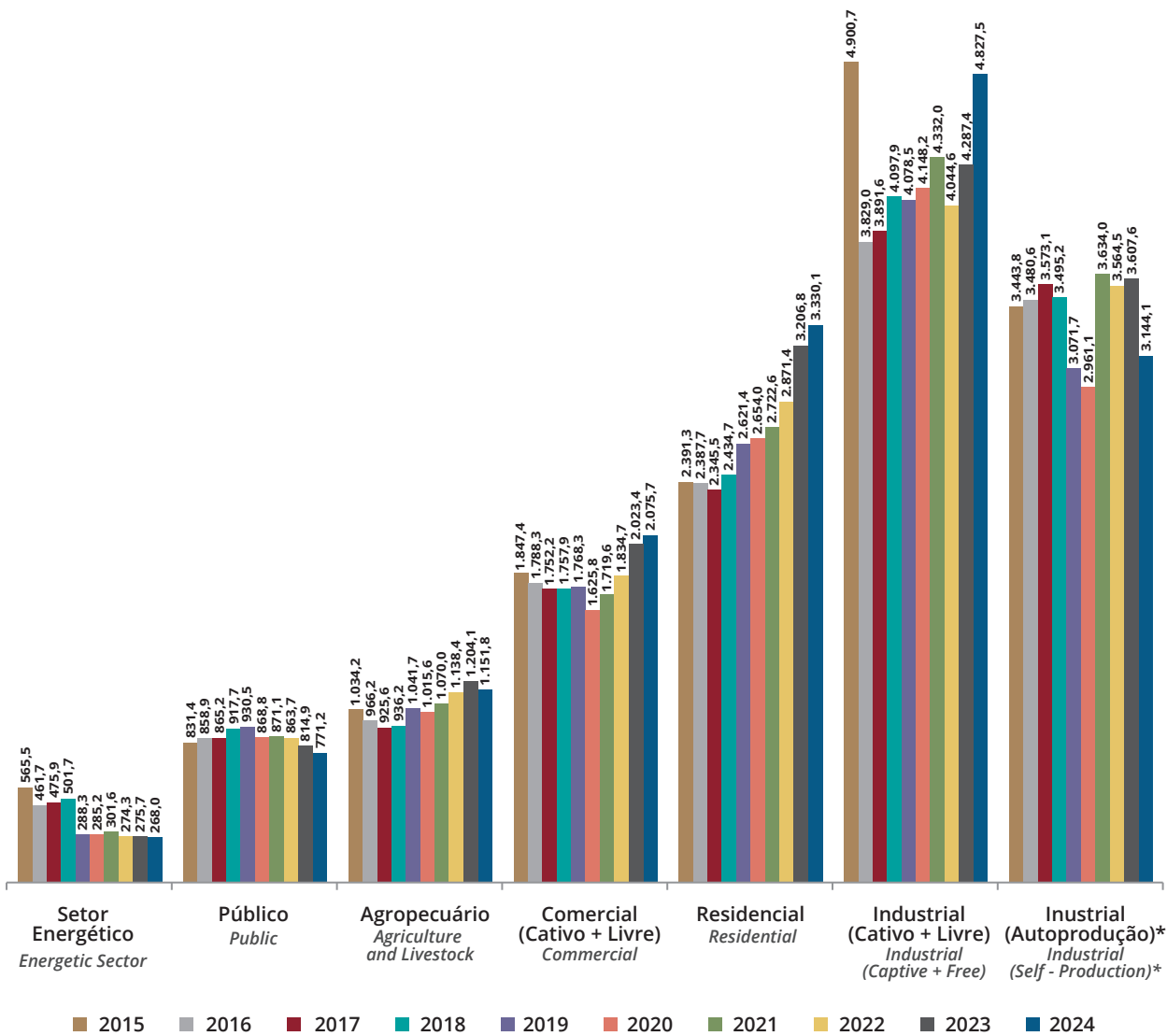
Gráfico 8.2.2 – Evolução do Consumo Final de Energia Elétrica no ES por Setor – Valores em GWh Graph 8.2.2 – Evolution of the Final Consumption of Electric Energy in the ES by Sector – Values in GWh
