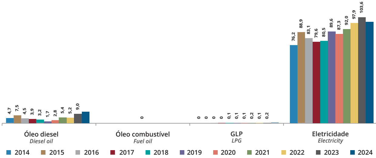
Gráfico 6.2.8 - Consumo Final Setor Agropecuário no ES por Fonte - Valores em mil tep Graph 6.2.8 - Final Consumption of the Agriculture and Livestock Sector in ES by Source - Values in thousand toe
