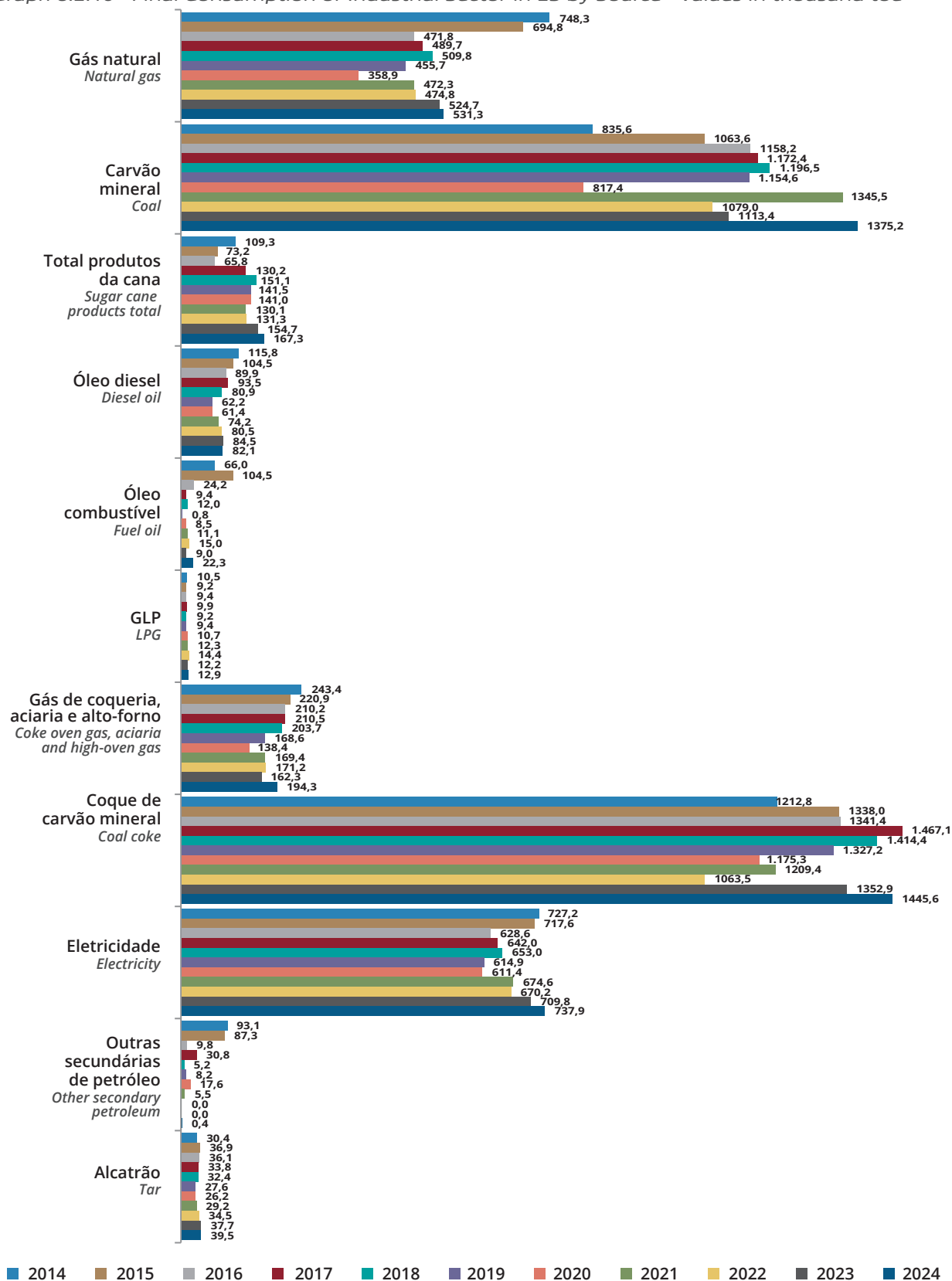
Gráfico 6.2.10 - Consumo Final Setor Industrial no ES por Fonte - Valores em mil tep
