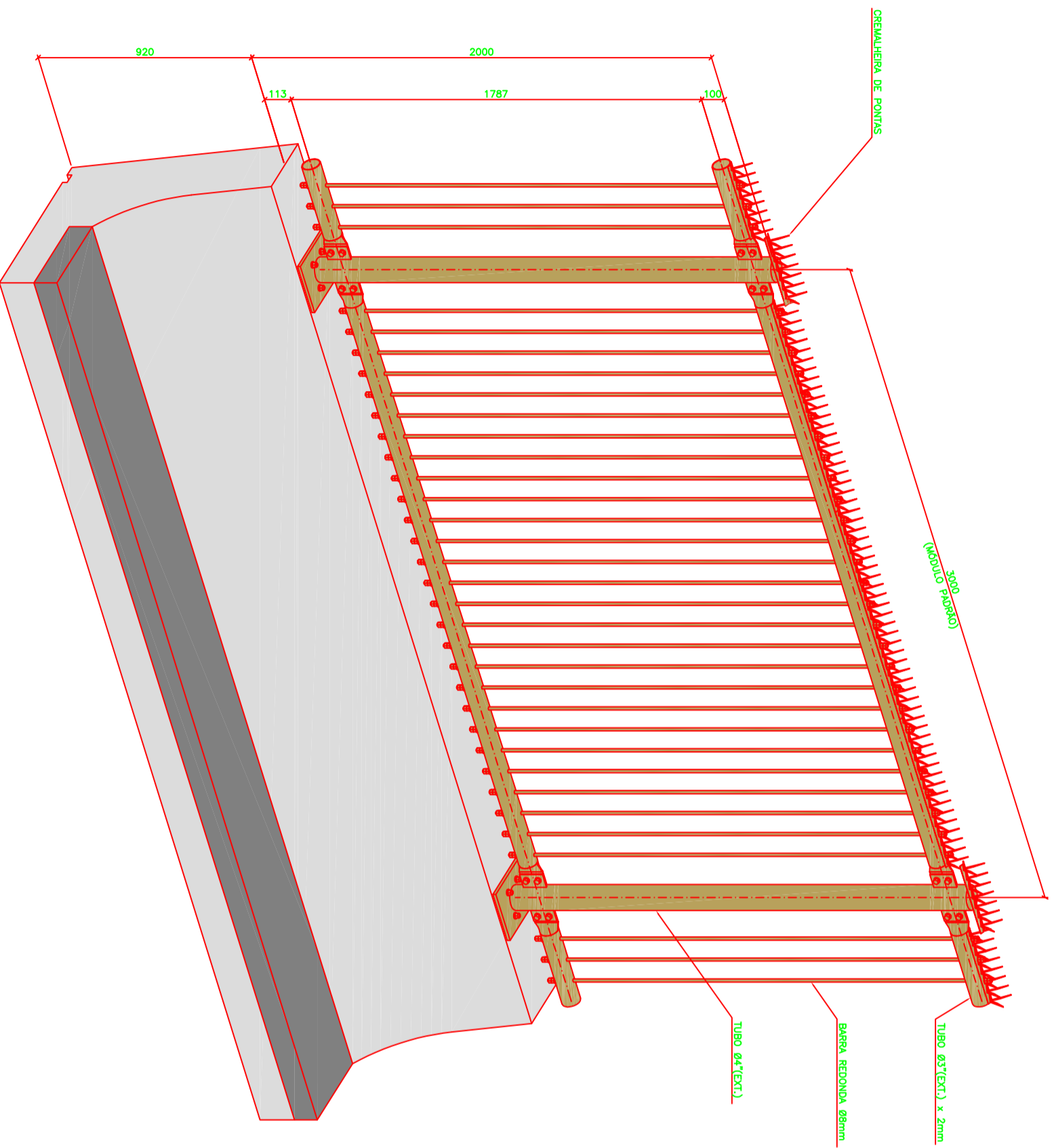
PERSPECTIVA ISOMÉTRICA ESQ:1:15
